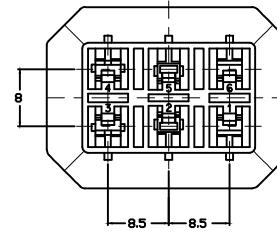
VIEW A-A
